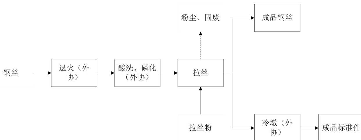
图 2-2 生产工艺流程图
