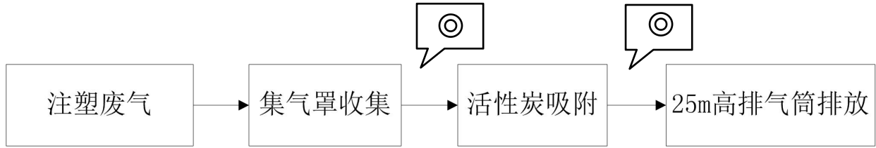
图 3-2 注塑废气处理工艺流程图
